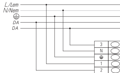
DALI EM (5 core cable) 5P
