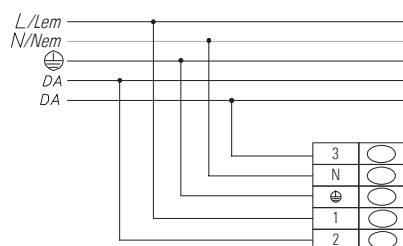
DALI EM (5 core cable) 5P 230 V
