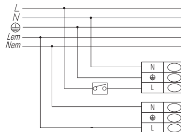
FO EM (5 core cable) 3P+3P 230 V
