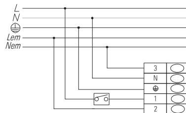
FO EM (5 core cable) 5P 230 V
