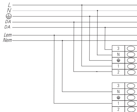
DALI EM (5+5core cable) 5P+5P 230 V
