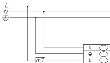
FO (3 core cable) 3P
