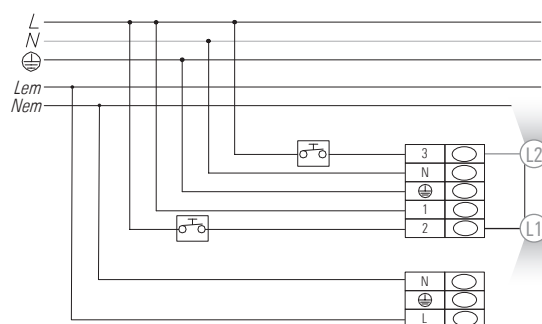
TD EM - double switch (5+3 core cable) 5P+3P
