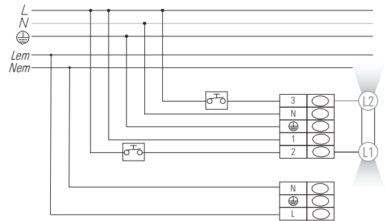
TD EM - double switch (5+3 core cable) 5P+3P 230 V
