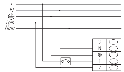
FO EM (5 core cable) 5P 230 V
